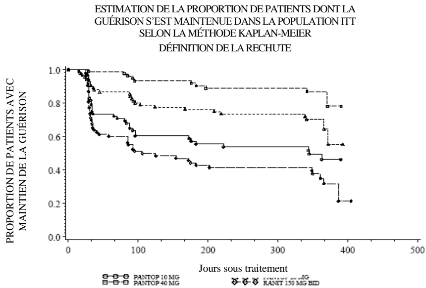
Courbe de l'analyse de Kaplan-Meier; 3001A1-303-US
