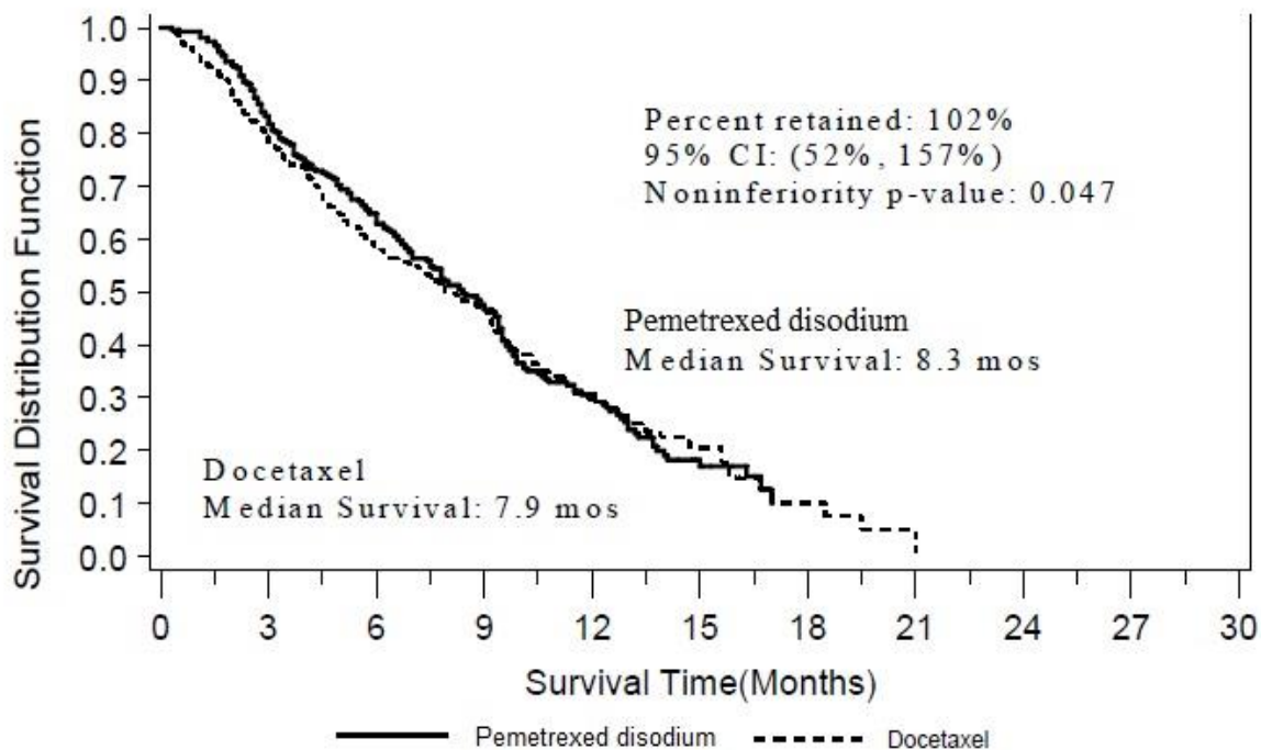
Figure 10 : Courbes de survie avec pemetrexed disodique par rapport au docétaxel (méthode de Kaplan-Meier)
