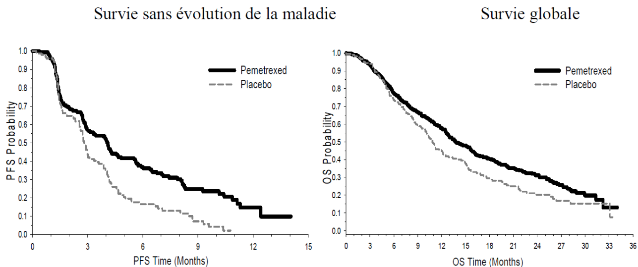
Figure 8: Traitement d'entretien après un traitement d'induction par pemetrexed disodique en association avec le cisplatine: Courbe de survie sans évolution de la maladie et de survie globale (méthode de Kaplan-Meier) pour pemetrexed disodique par rapport au placebo en présence de CPNPC non épidermoïde (valeur mesurée à partir de la randomisation)
