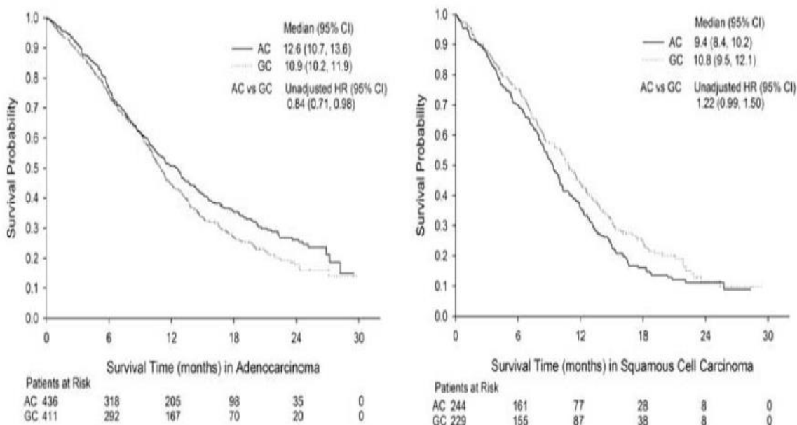
Figure 4: Courbes de survie globale de Kaplan-Meier pour Pemetrexed disodique –cisplatine (AC) contre gemcitabine-cisplatine (GC) dans le cancer du poumon non à petites cellules – Sousgroupes histologiques : Adénocarcinome et carcinome épidermoïde – Population ITT
