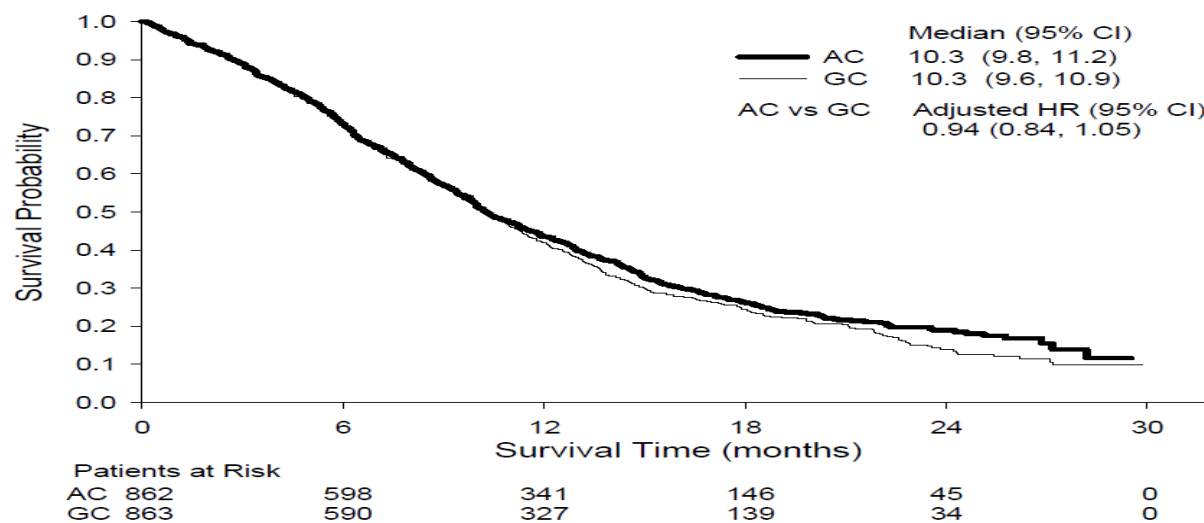
Figure 2: Courbes de survie globale de Kaplan-Meier pour l'association Pemetrexed disodique -cisplatine (AC) et l'association gemcitabine-cisplatine (GC) dans le cancer du poumon non à petites cellules – Population ITT
