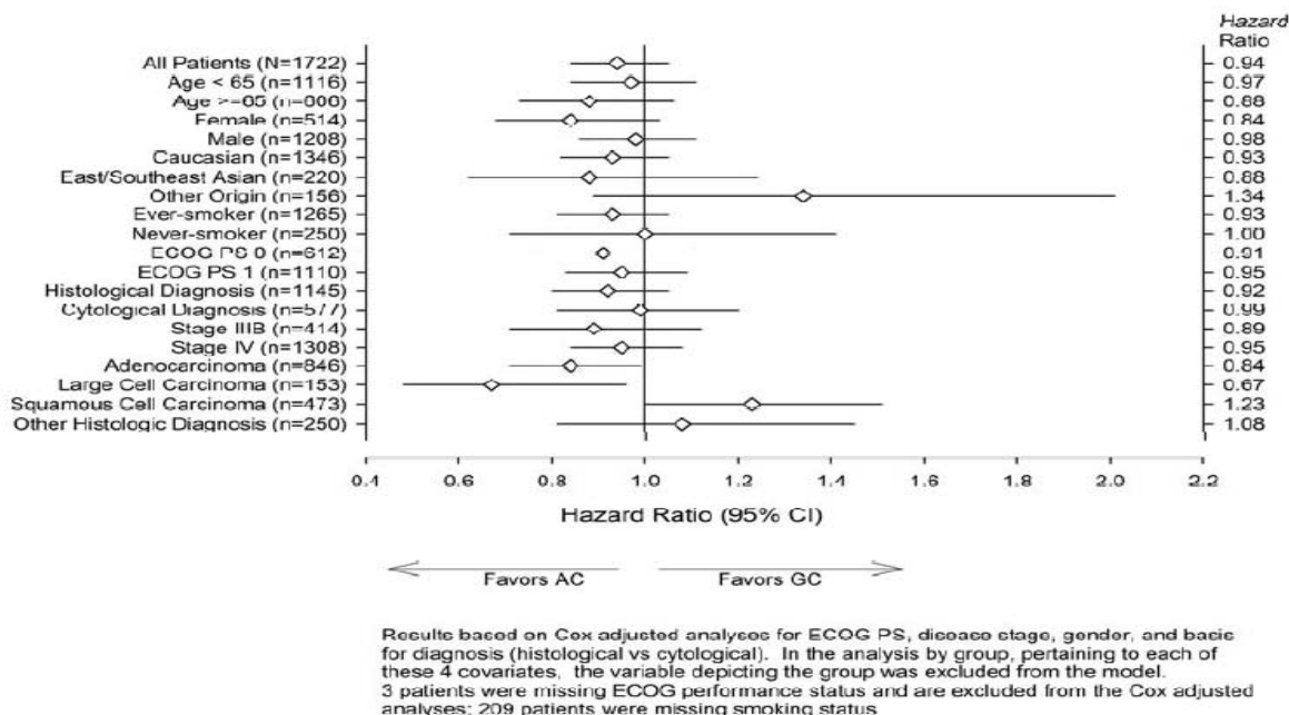
Figure 3: Graphique en forêt des rapports de risques ajustés de la survie globale des sousgroupes Pemetrexed disodique -cisplatine contre gemcitabine-cisplatine dans le cancer du poumon non à petites cellules – Population ITT
