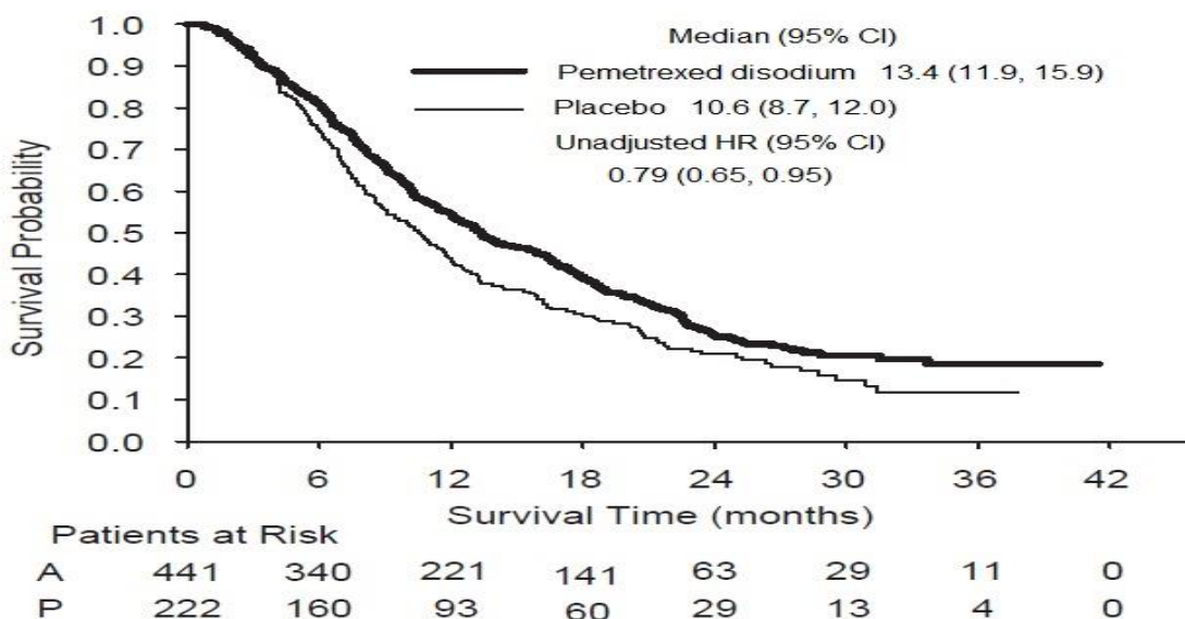
Figure 5: Courbes de survie globale de Kaplan-Meier pour Pemetrexed disodique (A) par rapport au placebo (P) dans le CPNPC – Population ITT
