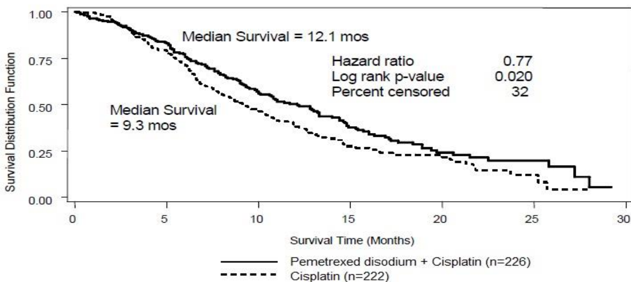
Figure 1 : Courbes de survie (méthode de Kaplan-Meier)
