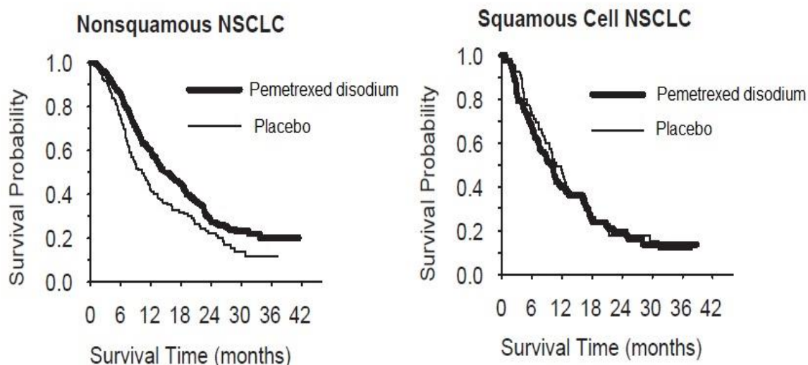
Figure 6 : Courbes de survie globale de Kaplan-Meier pour Pemetrexed disodique par rapport au placebo dans le CPNPC - CPNPC non épidermoïde et CPNPC épidermoïde
