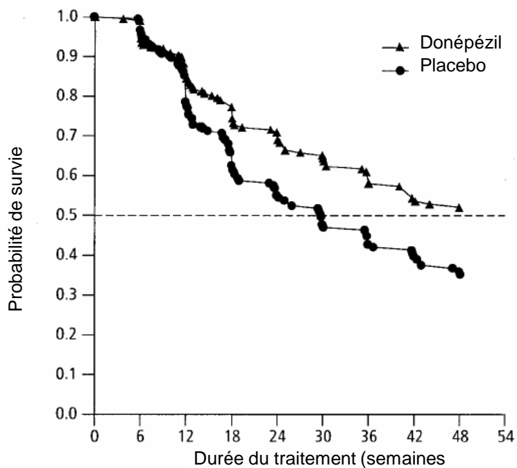
Figure 3 – Courbes de survie (temps écoulé avant une détérioration manifeste sur le plan clinique de la capacité fonctionnelle) dans les 2 groupes observés
