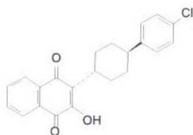
Atovaquone
