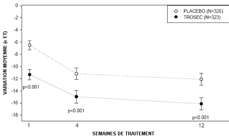
Figure 5 – Variation moyenne des épisodes d'incontinence d'urgence/semaine à partir des valeurs de départ, par visite : étude 2
