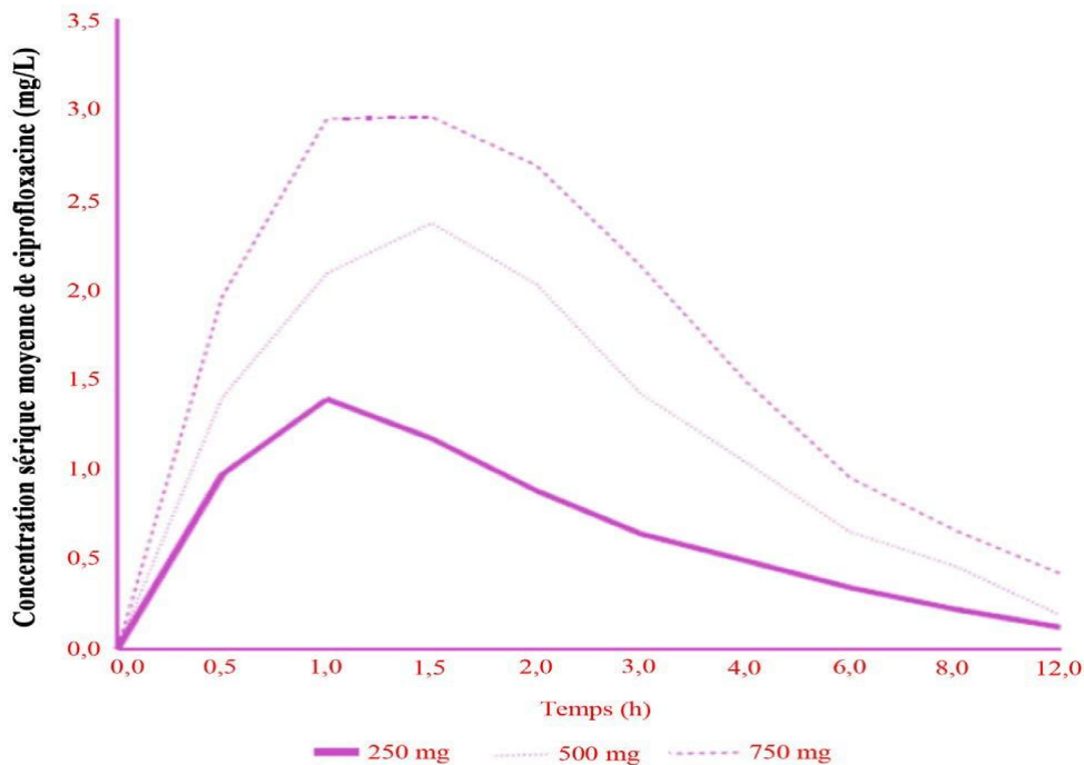
Figure 1 : Concentrations sériques moyennes de ciprofloxacine après une administration orale unique
