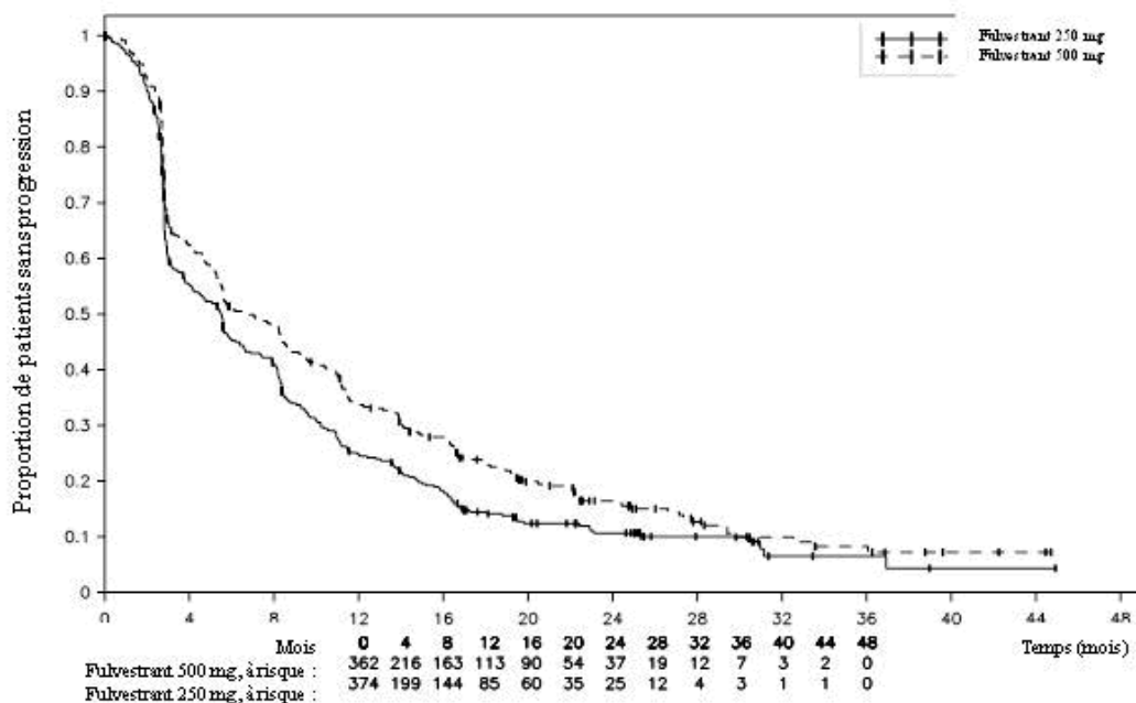
Figure 9 Essai CONFIRM (D6997C00002) – Courbes de Kaplan-Meier de la survie sans progression – Sujets inclus : toutes les patientes randomisées pour recevoir 500 mg de fulvestrant ou à 250 mg de fulvestrant
