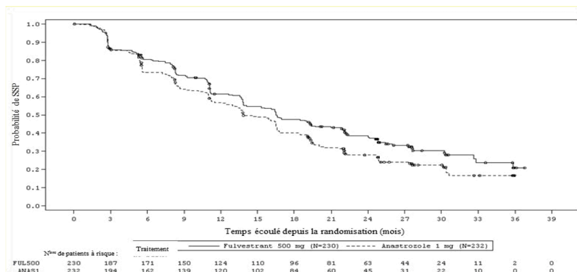
Figure 6 Courbe de Kaplan-Meier de la survie sans progression (évaluation par le chercheur, population en IDT) – Étude FALCON
