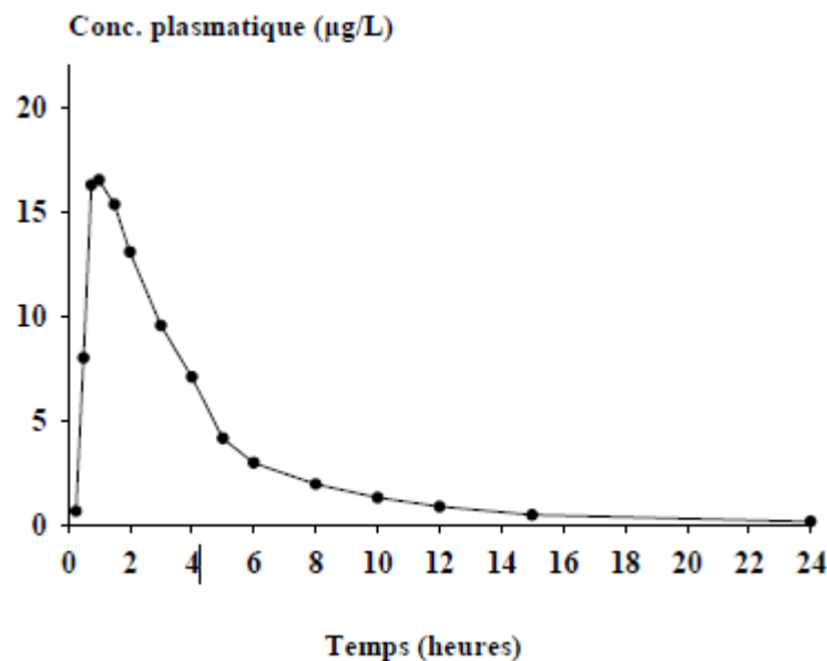
Figure 1 : Courbe des concentrations plasmatiques moyennes produites par une dose de 20 mg de vardénafil en comprimés administrée par voie orale
