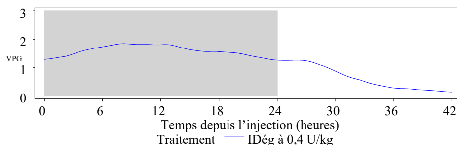
Figure 1-1 : Profil de la vitesse de perfusion du glucose moyenne (état d'équilibre) avec Tresiba® à 0,4 U/kg chez les patients atteints de diabète sucré de type 1
