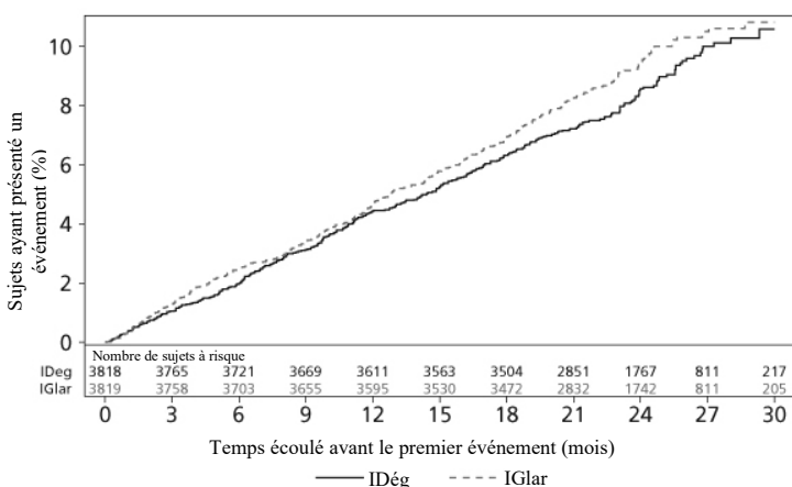
Figure 2-3 : Probabilité d'événements cumulatifs pour le temps écoulé avant le premier ECIM confirmé par le CEE dans l'essai DEVOTE
