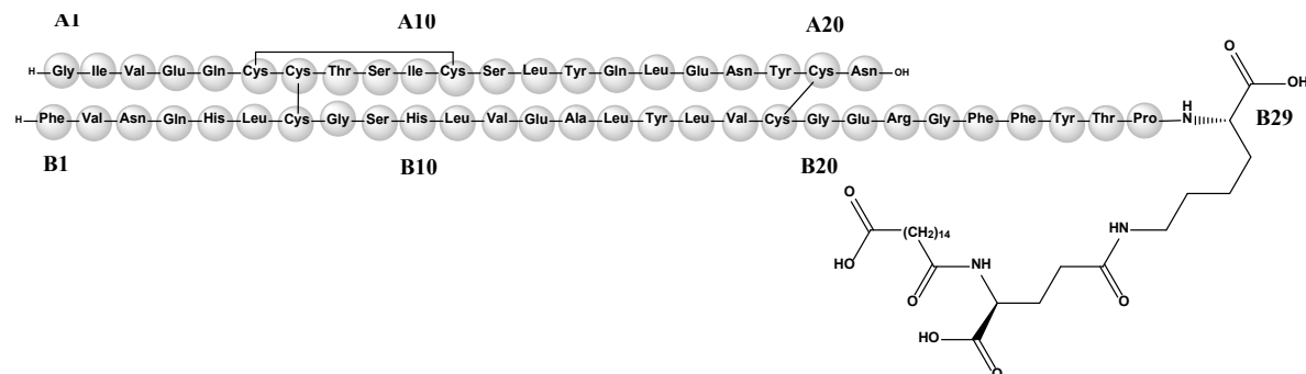
Figure 2-1 : Formule de structure de l'insuline dégludec
