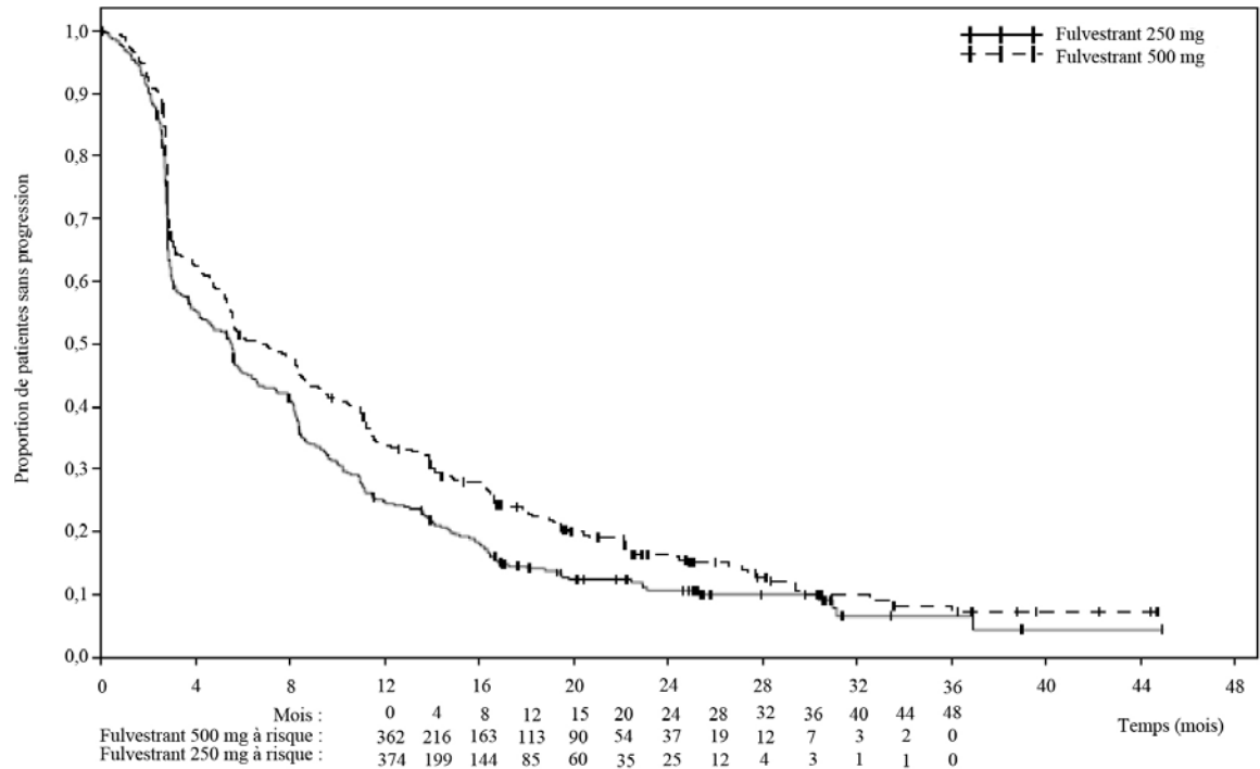
Figure 9. Essai CONFIRM (D6997C00002) – Courbes de Kaplan-Meier de la survie sans progression – Sujets inclus : toutes les patientes réparties aléatoirement
