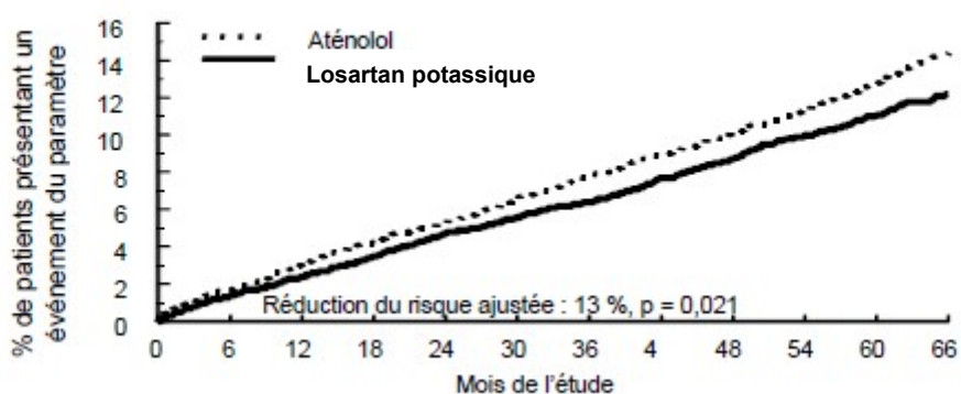
Figure 1 – Courbe de Kaplan-Meier (observation) — Composantes regroupées du paramètre principal
