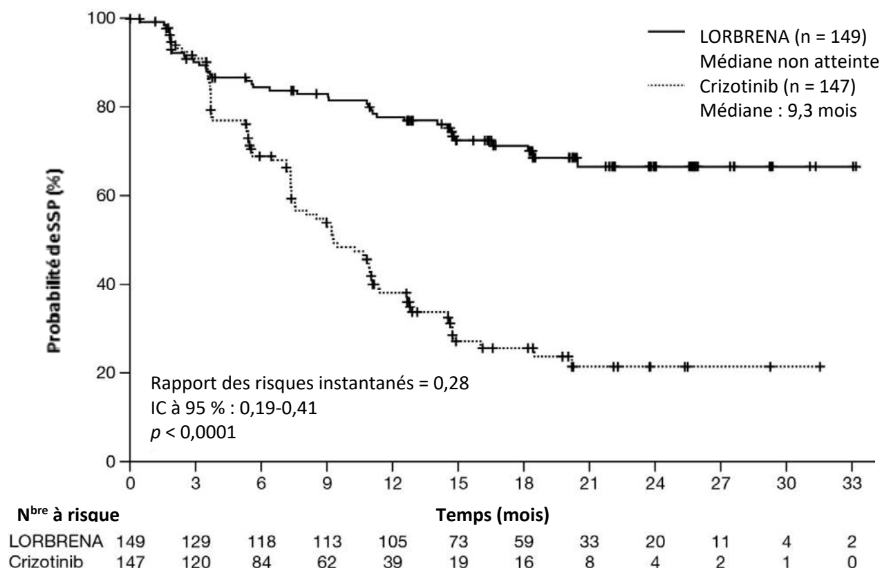
Figure 1. Courbe de Kaplan-Meier relative à la survie sans progression déterminée par une ECII lors de l'étude de phase III B7461006
