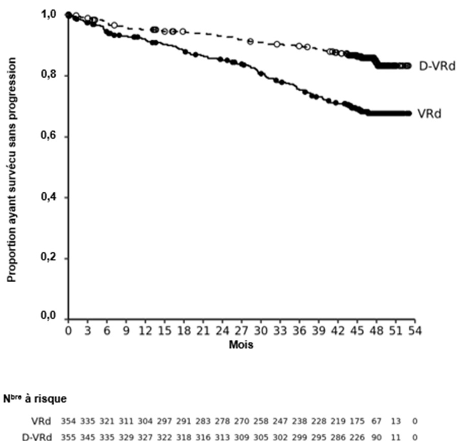
Figure 1 : Courbe de Kaplan-Meier pour la survie sans progression (SSP) dans l'étude MMY3014
