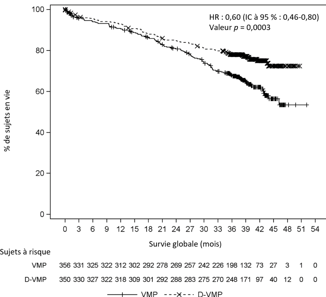
Figure 5 : Courbe de Kaplan-Meier pour la survie globale; ensemble d'analyse en intention de traiter dans l'étude MMY3007
