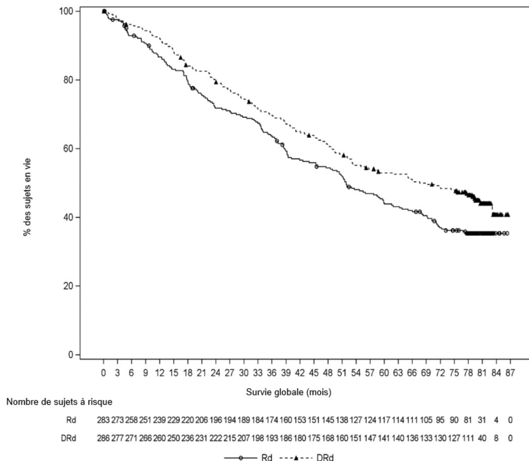
Figure 7 : Courbe de Kaplan-Meier pour la survie globale (SG) dans l'étude MMY3003 (population en IDT)
