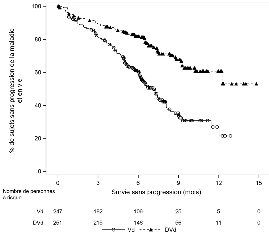
Figure 8 : Courbe de Kaplan-Meier pour la survie sans progression dans l'étude MMY3004 (suivi médian de 7,4 mois)
