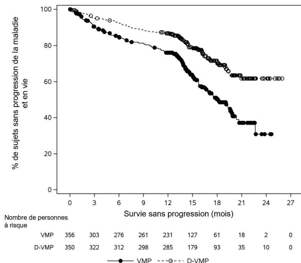
Figure 4 : Courbe de Kaplan-Meier pour la survie sans progression dans l'étude MMY3007 (suivi médian de 16,5 mois)
