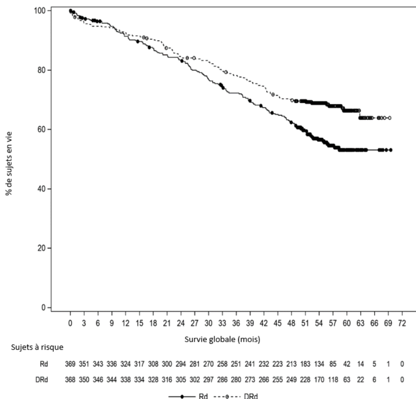
Figure 3 : Courbe de Kaplan-Meier pour la survie globale (SG) dans l'étude MMY3008 (population en IDT)
