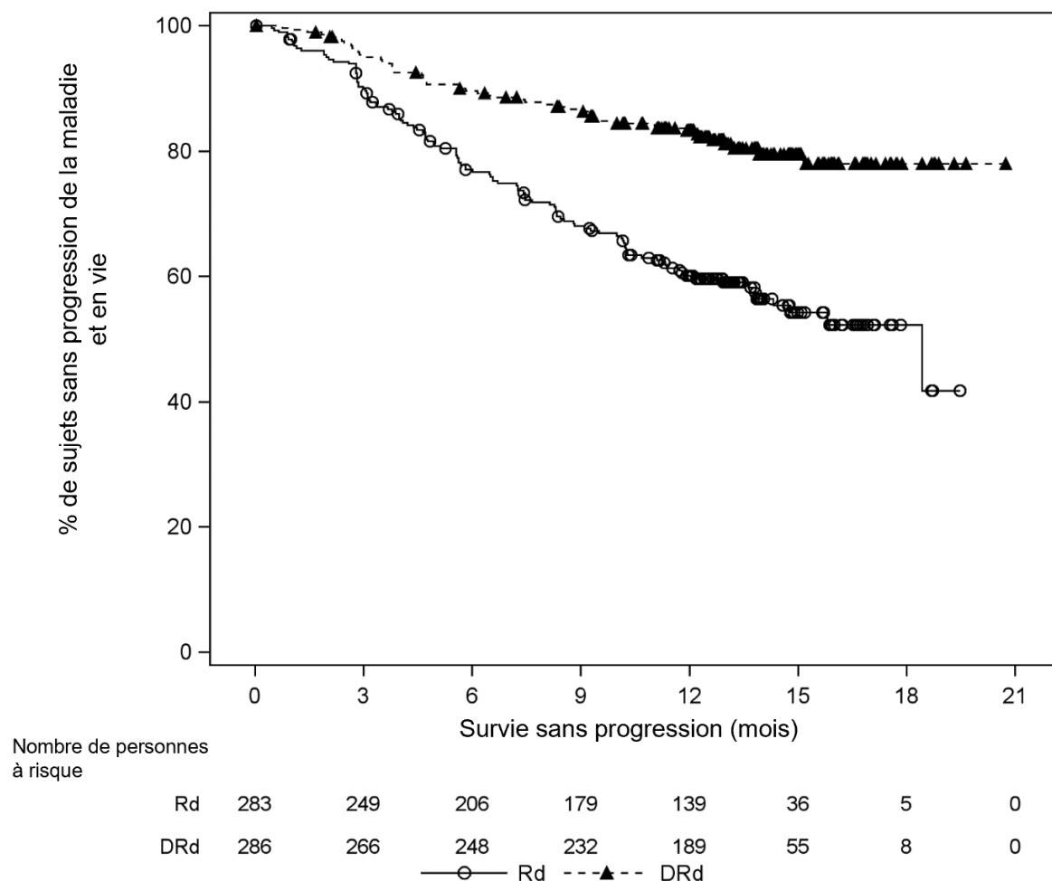
Figure 6 : Courbe de Kaplan-Meier pour la survie sans progression dans l'étude MMY3003 (suivi médian de 13,5 mois)
