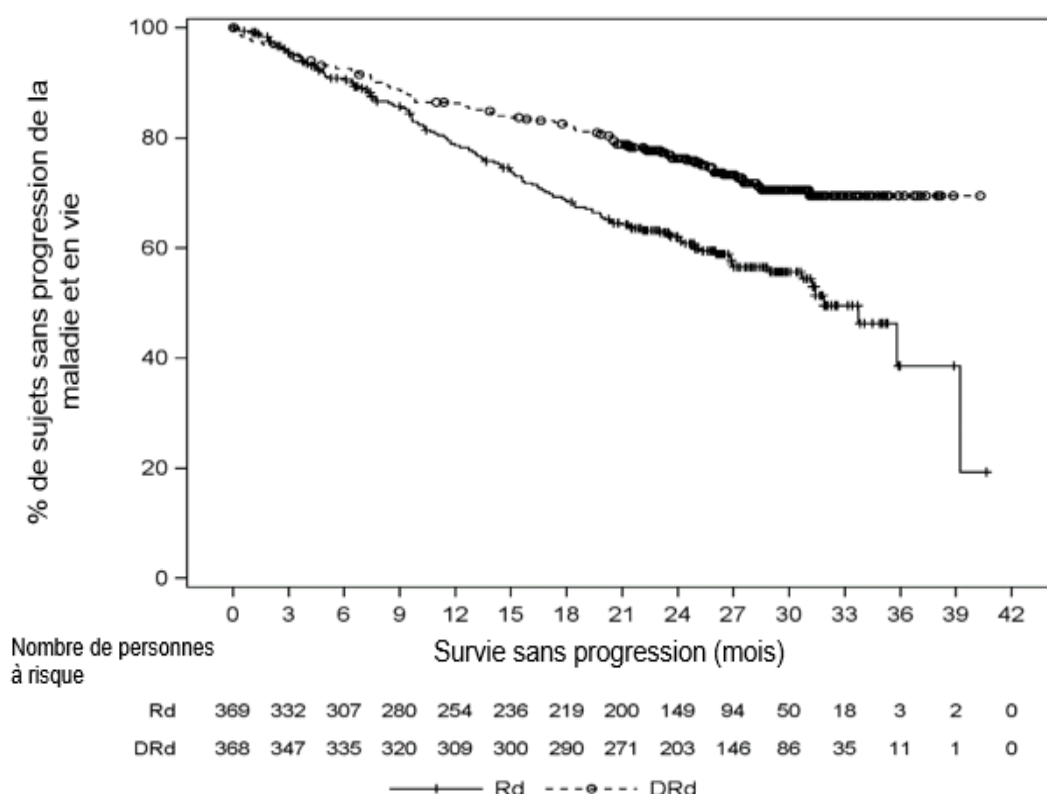
Figure 2 : Courbe de Kaplan-Meier pour la survie sans progression dans l'étude MMY3008 (analyse principale)
