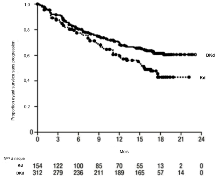
Figure 11 : Courbe de Kaplan-Meier de la SSP dans l'étude CANDOR
