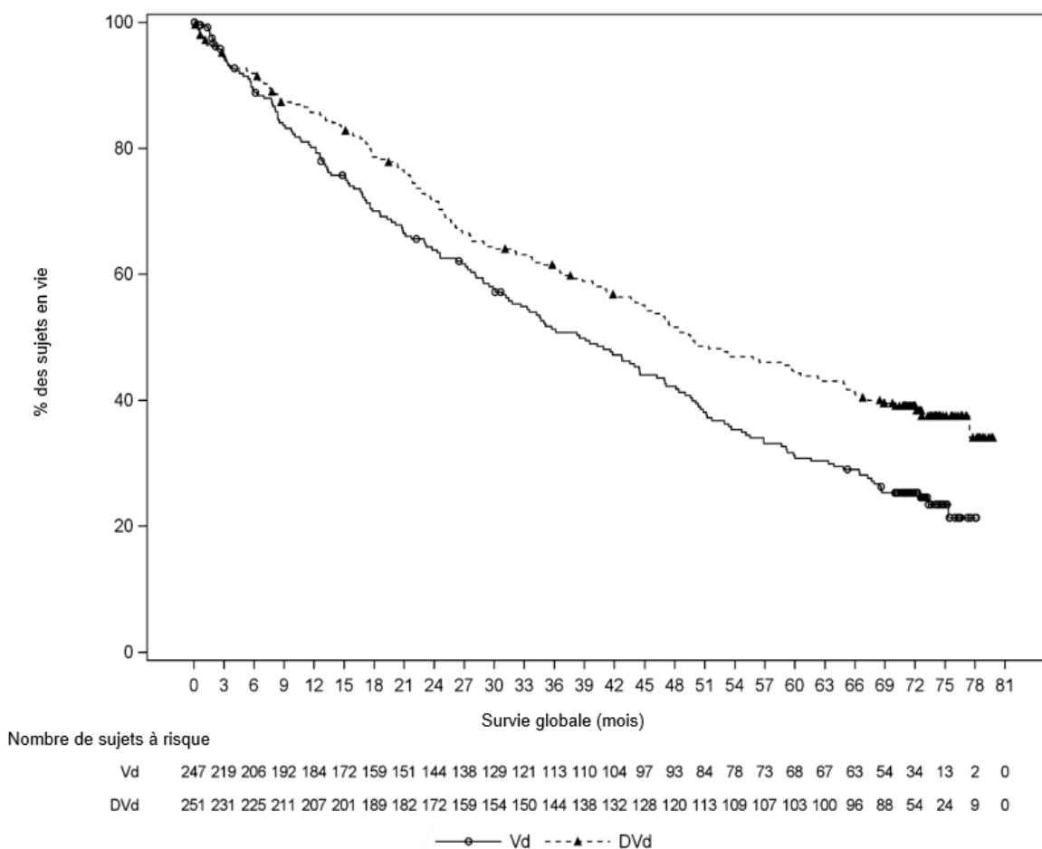
Figure 9 : Courbe de Kaplan-Meier pour la survie globale (SG) dans l'étude MMY3004 (population en IDT)
