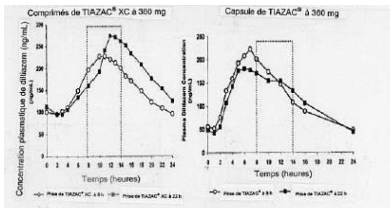
Figure 1: Évolution de la concentration plasmatique de diltiazem durant 24 heures à l'état d'équilibre 1
