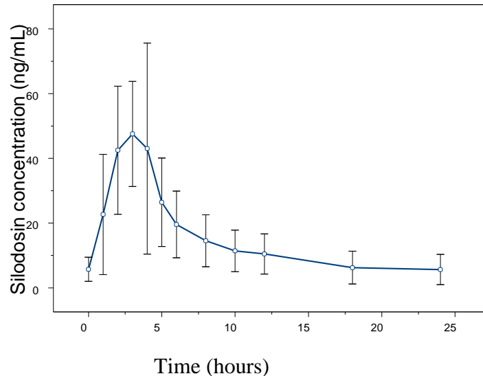
Figure 1 Profil de la concentration plasmatique moyenne ( \pm ET) en silodosine à l'état d'équilibre en fonction du temps chez des sujets de sexe masculin en santé appartenant à la tranche d'âge visée après la prise de 8 mg de silodosine, une fois par jour, avec de la nourriture
